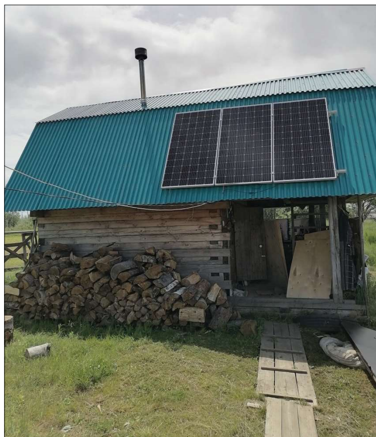
Солнечная панель на крыше
